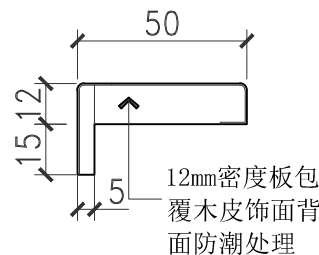
门套线大样图
