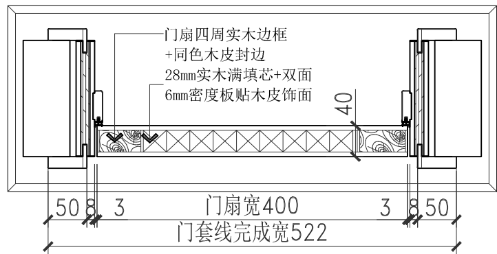
N型门扇小样横剖图
