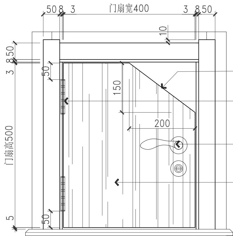
N型门扇小样立面图
