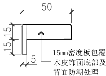
门套线大样图
